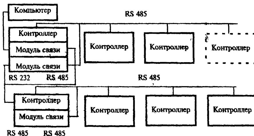
Рисунок 5 - Примерная структурная схема построения СКУД 4-го класса с несколькими ветвями
